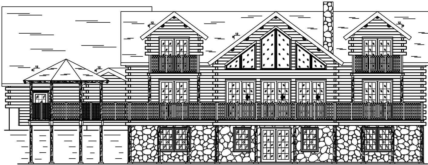
ELEVATION A
