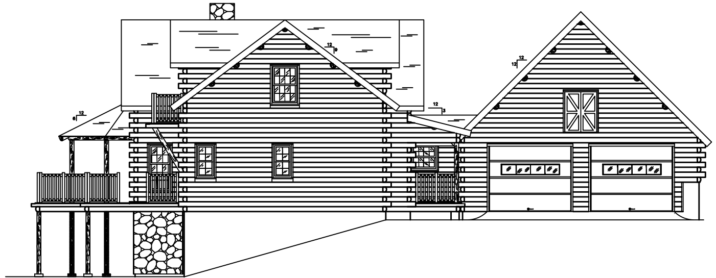
ELEVATION B
