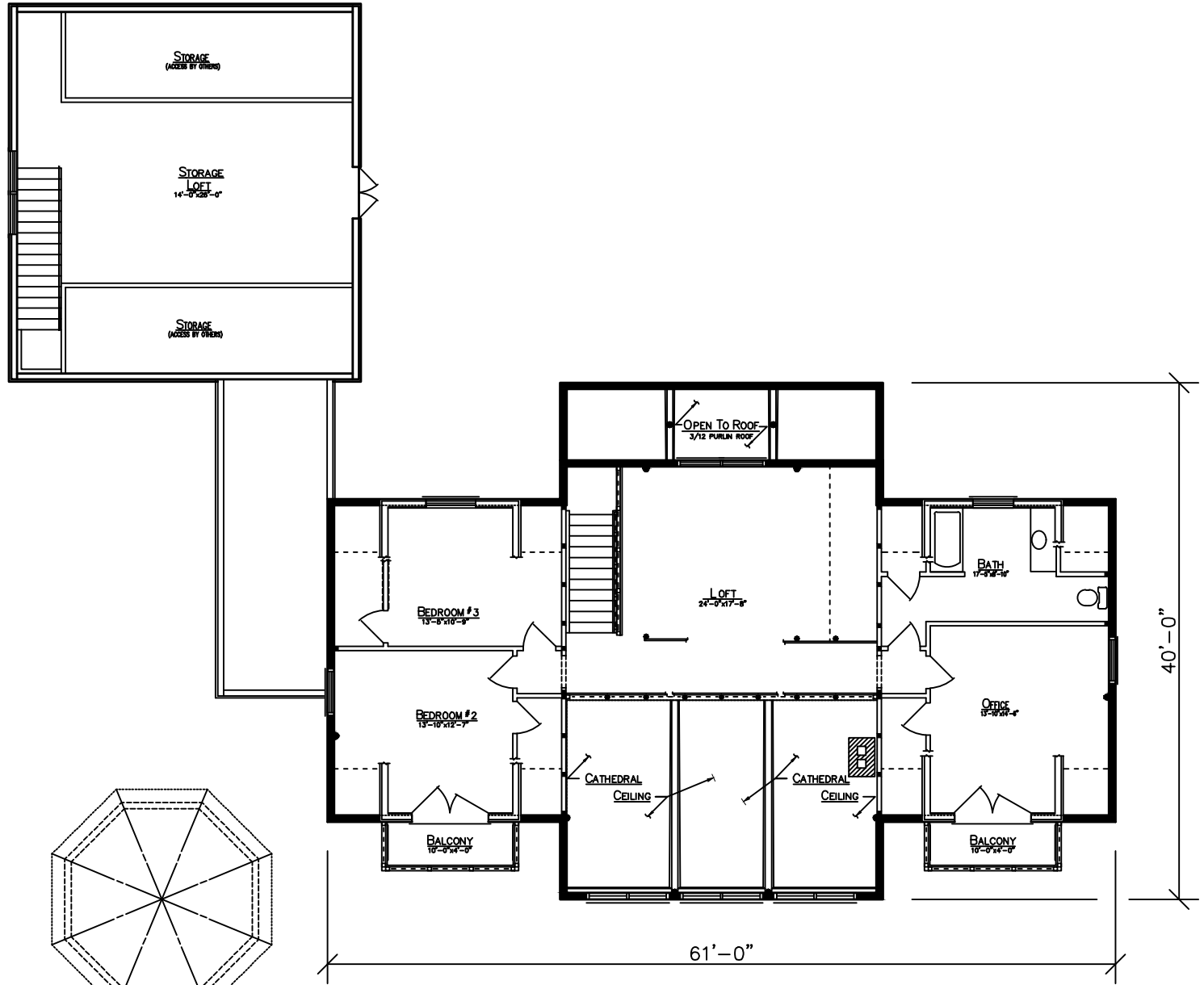
LOFT PLAN
