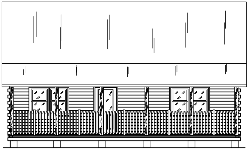
ELEVATION A
