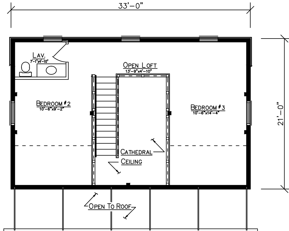
LOFT PLAN
